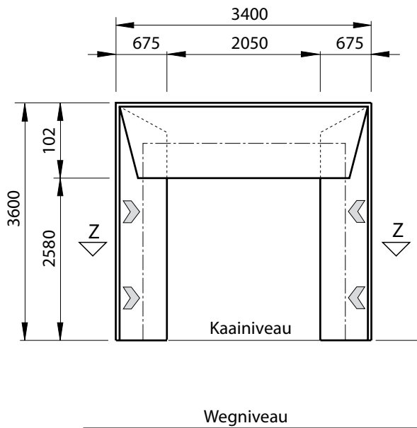
Schema van het model WS574-34x36-P600
